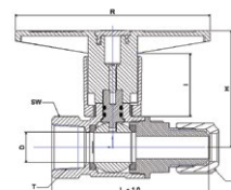
ברז כדורי דגם S.H.N.F. תברג פנים חיבור לצינור נחושת פלייר
