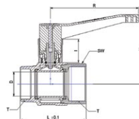
ברז כדורי דגם S.H.A. תברג פ.ח. קנה גבוה
