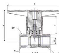
ברז כדורי דגם S.H.N. תברג פ.פ. קנה גבוה
