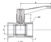
ברז כדורי דגם S.H.N. תברג פ.פ. קנה גבוה
