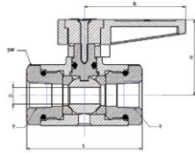
דגם S.M.N. תבריג פנים פנים ברז למנומטר עם חריר שחרור פ.פ.
