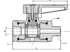
דגם S.M.A. תבריג פנים חוץ ברז למנומטר עם חריר שחרור פ.ח.
